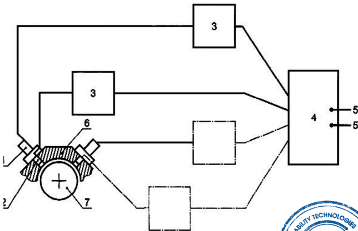
Рисунок С.3 - Схема системы измерений абсолютного движения с использованием датчиков бесконтактного и инерционного типов
