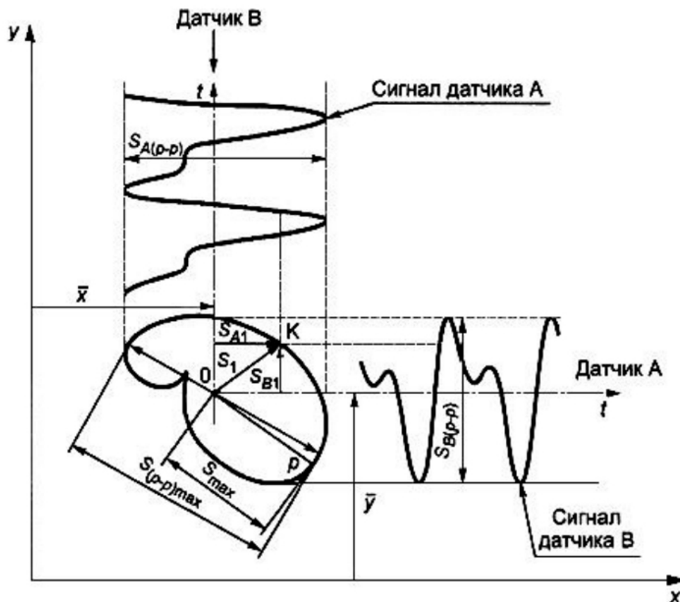
Рисунок В.2 - Сигналы вибрации, соответствующие определенной траектории движения вала
